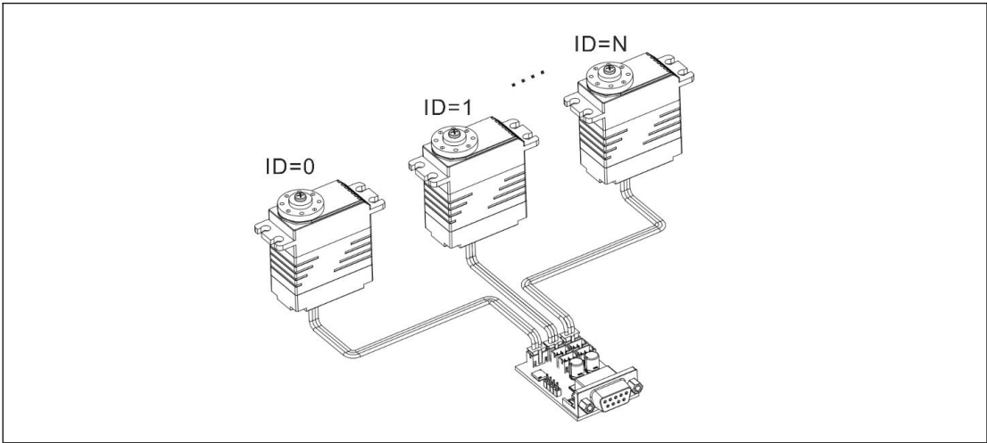
并联
