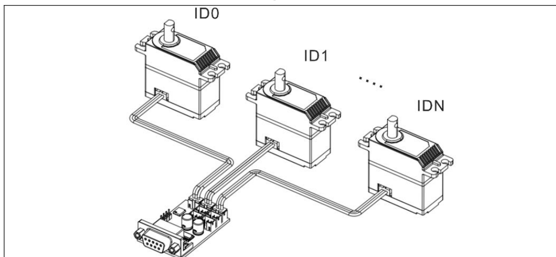
并联
